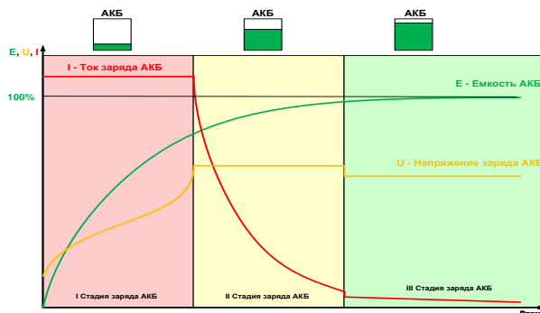
Рисунок 4.5.1 (Процесс зарядки аккумуляторной батареи).
